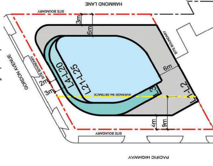
25 storeys (79m)
